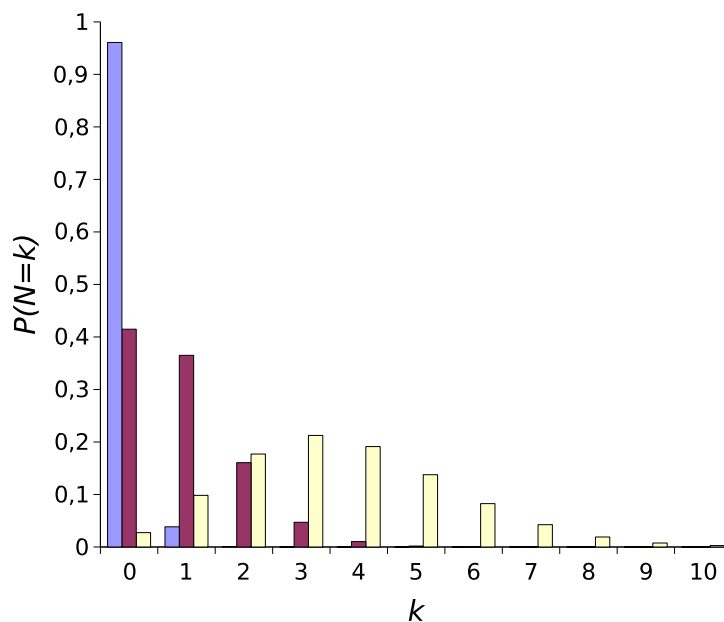
FIG. 1 – Distribution de la loi de Poisson pour les intensités \lambda = 0,04 (bleu), \lambda = 0,88 (rouge) et \lambda = 3,6 (jaune).
